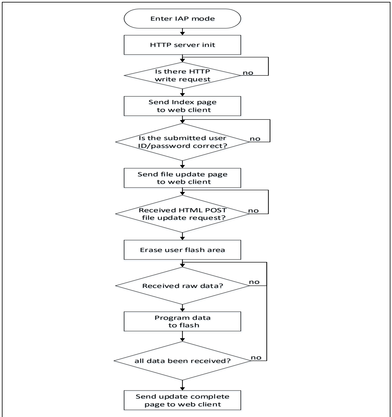
图 10 使用 HTTP 实现 IAP 的流程图
