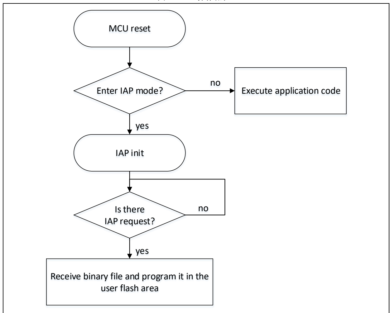
图 1 IAP 操作流程
