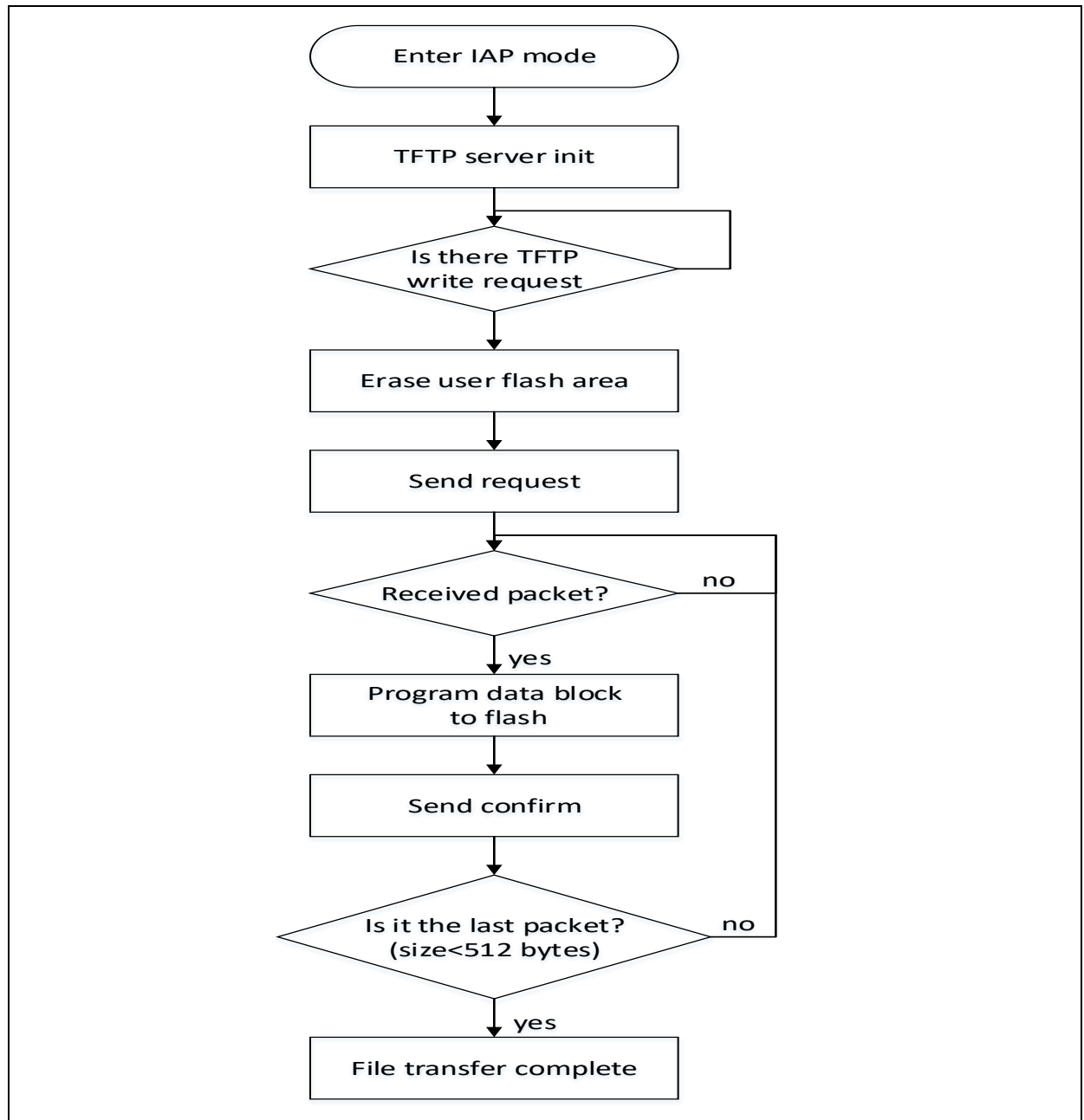
图 3 使用 TFTP 实现 IAP 流程图
