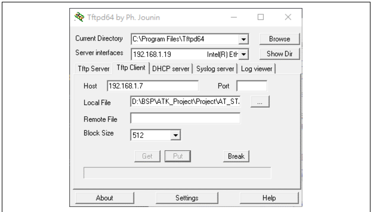
图 4 TFTP64 对话框
