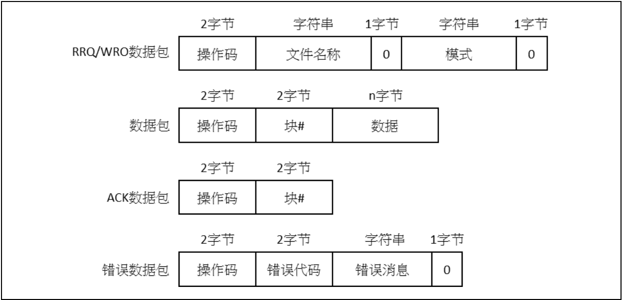
图 2 TFTP 数据包
