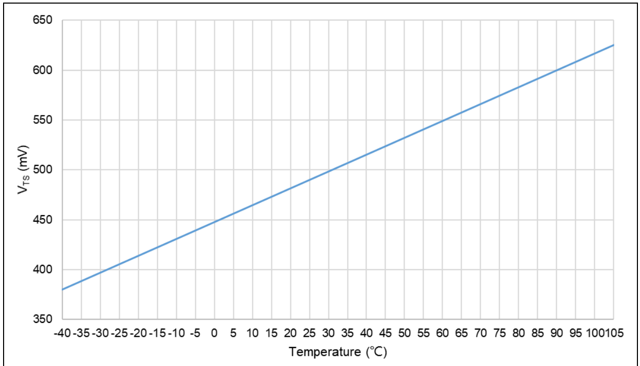
图 2. AT32F402 V_{TS} 对温度理想曲线图
