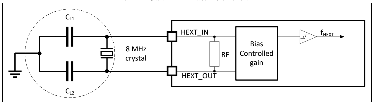
图 13. 使用 8 MHz 晶体的典型应用
