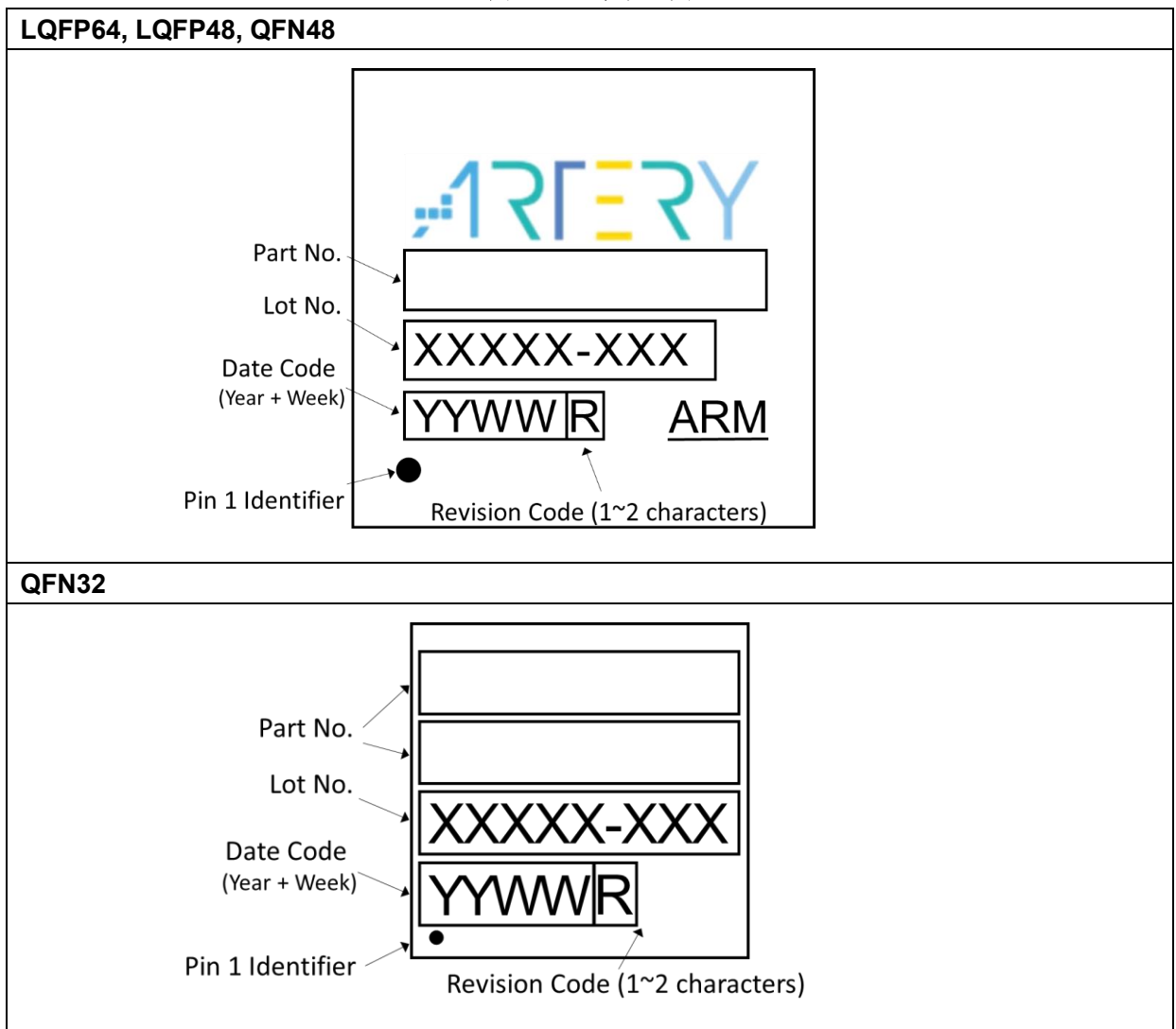
图 36. 丝印示意图
