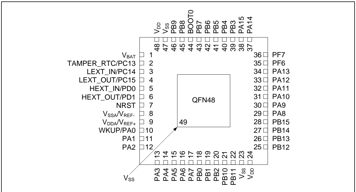
图 4. AT32F415 系列 QFN48 引脚分布
