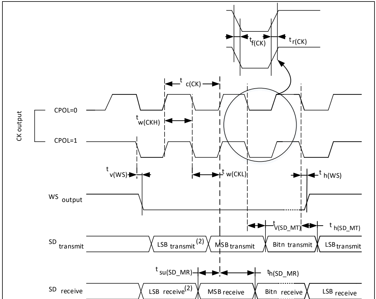
图 23. I 2 S 主模式时序图 (Philips 协议)
