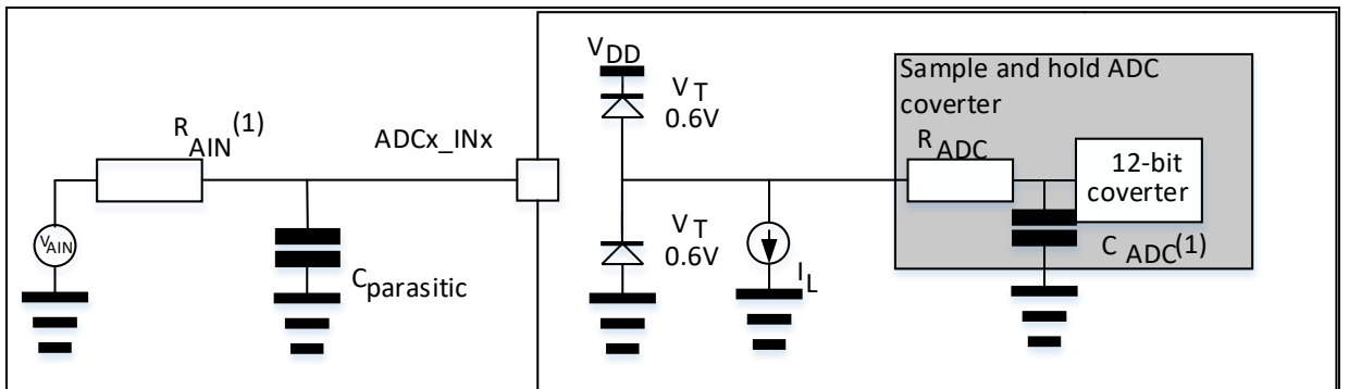
图 28. 使用 ADC 典型的连接图
