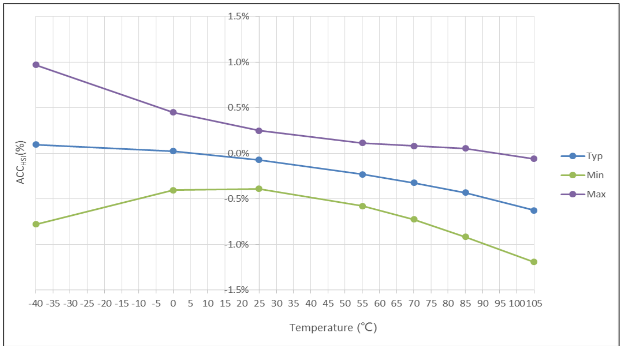
图 17. HICK 时钟精度与温度的对比
