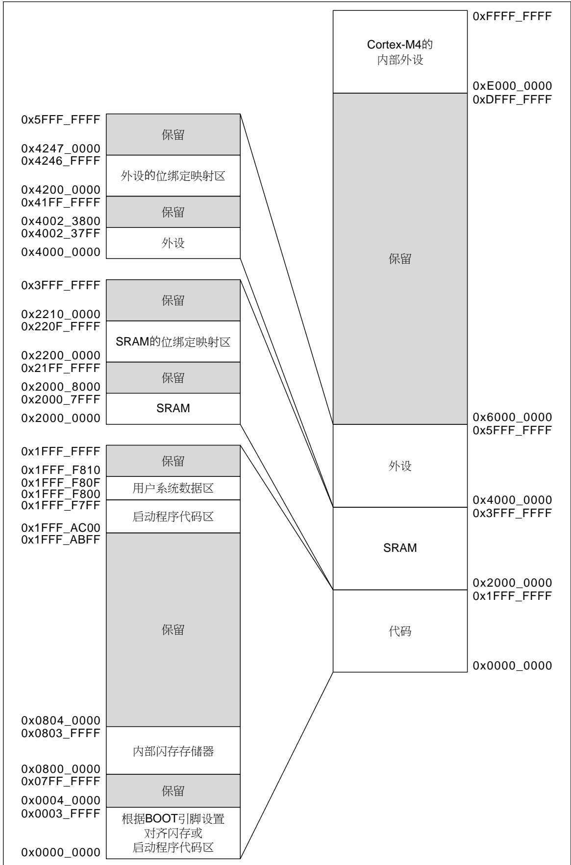
图 6. 存储器图
