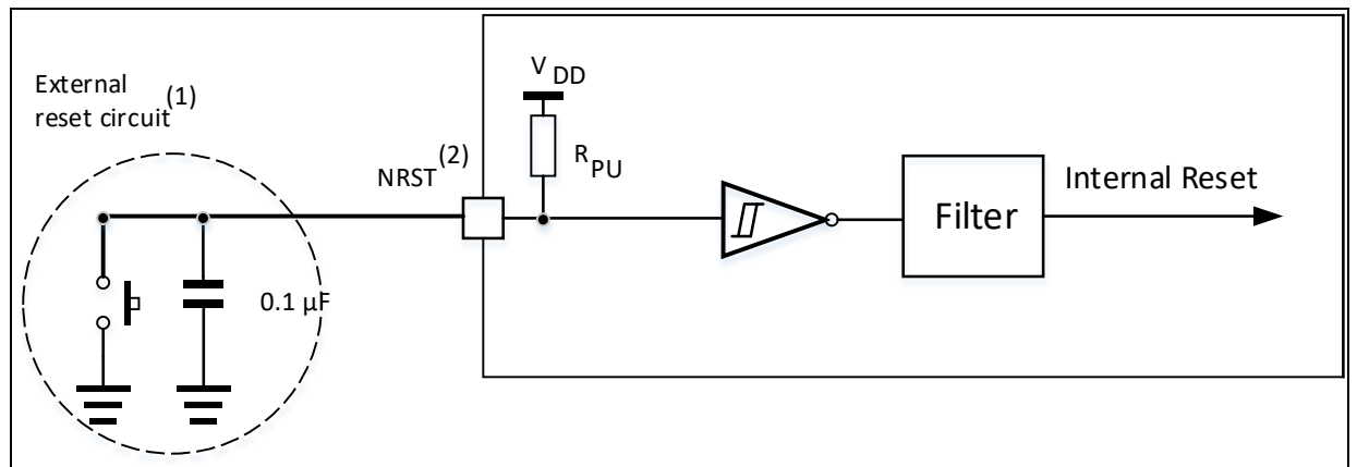
图 18. 建议的 NRST 引脚保护
