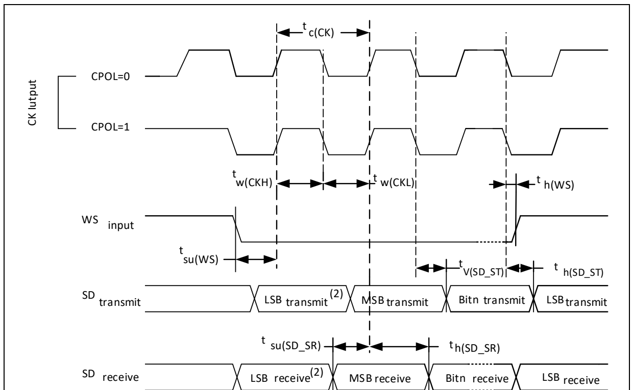
图 22. I 2 S 从模式时序图 (Philips 协议)
