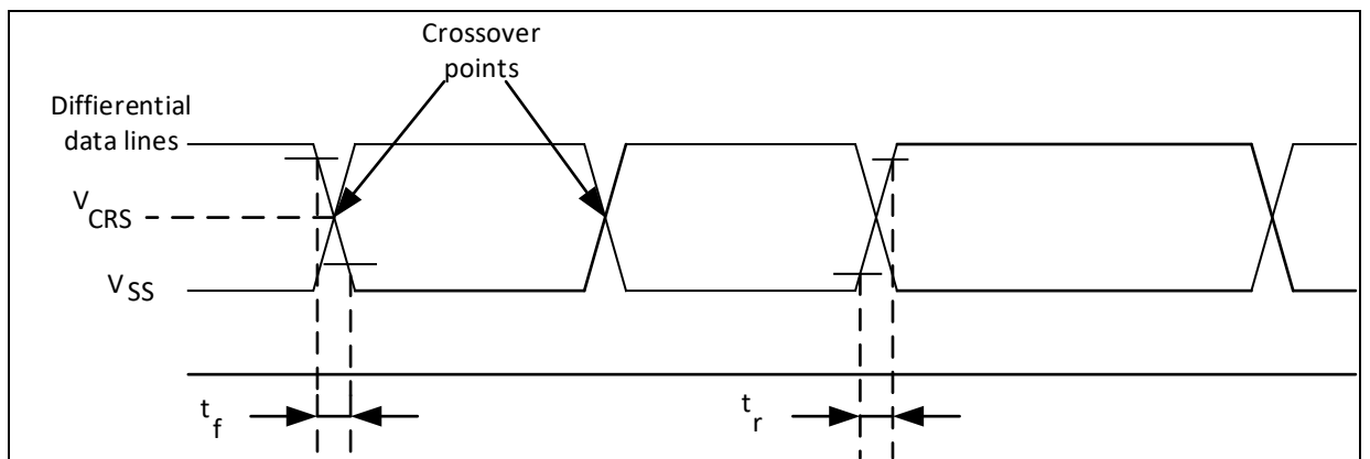
图 26. OTGFS 时序：数据信号上升和下降时间定义
