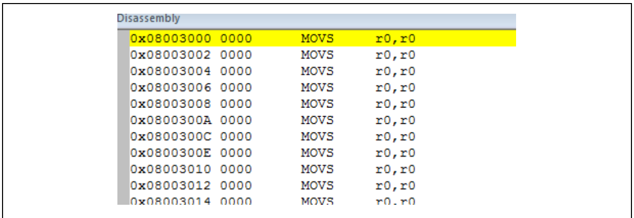
图 38. 代码查看
