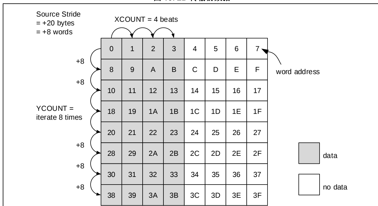
图 13. 2D 传输前数据
