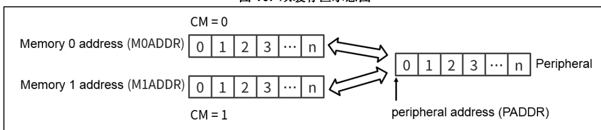
图 10. 双缓存区示意图
