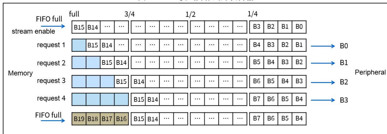
图 4. FIFO 模式内存到外设传输
