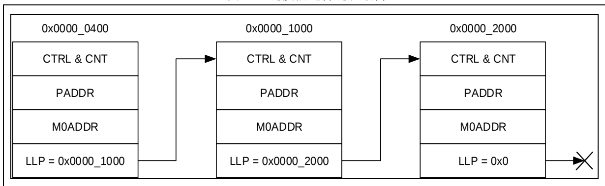
图 12. 链接描述符链表结构
