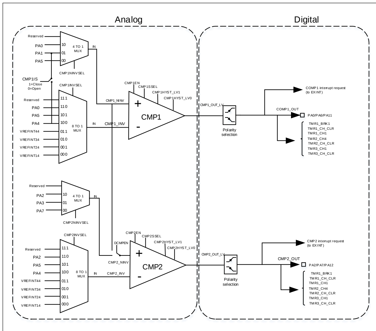
图 1. CMP 功能框图
