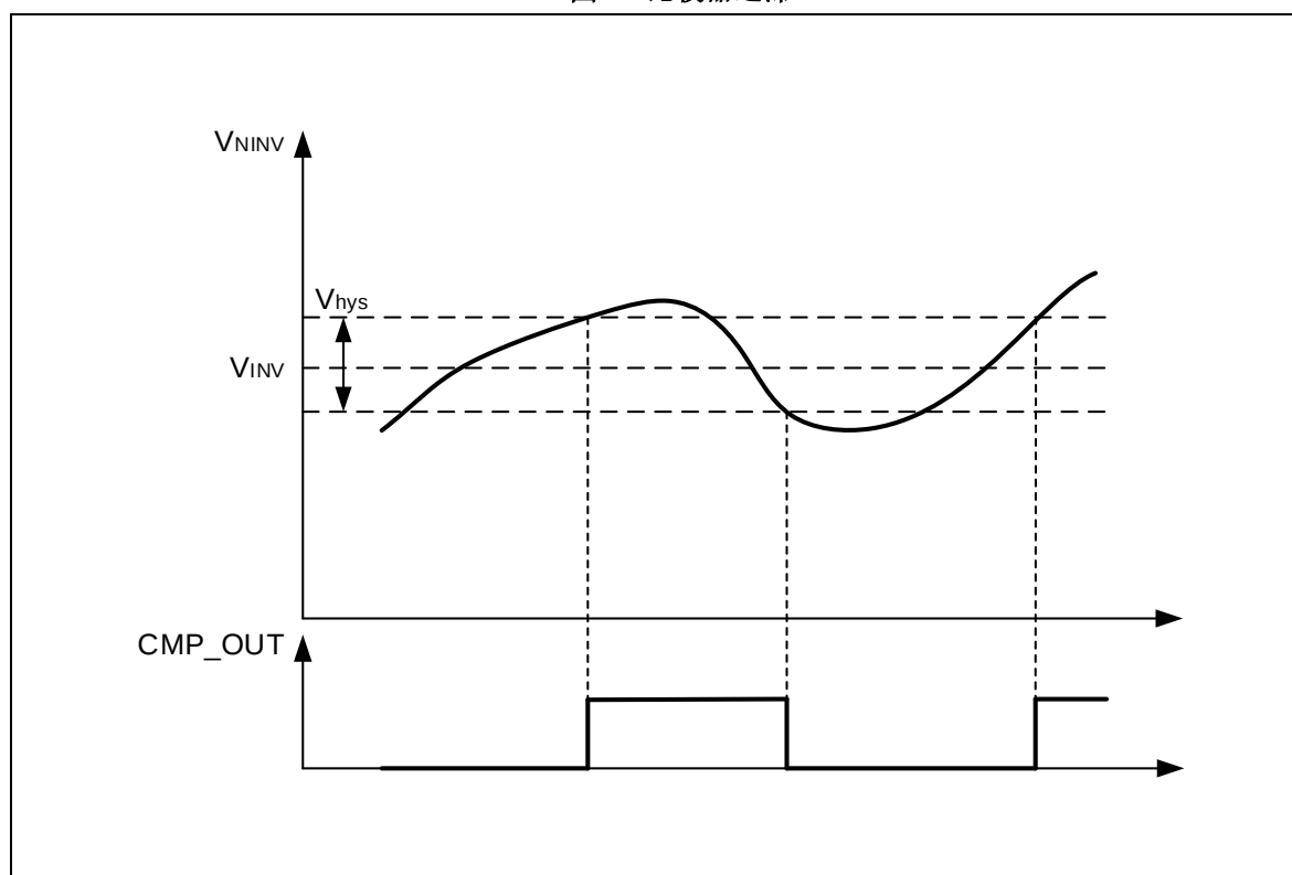
图 2. 比较器迟滞
