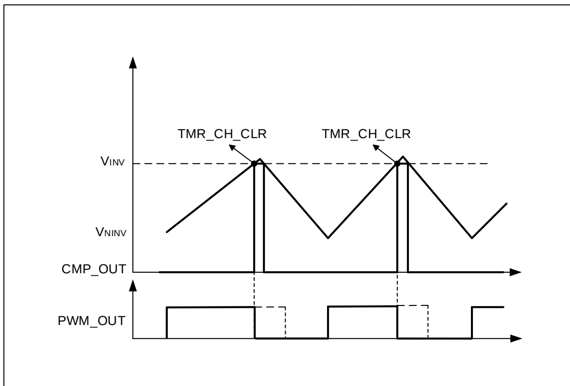
图 3. 逐周期电流控制
