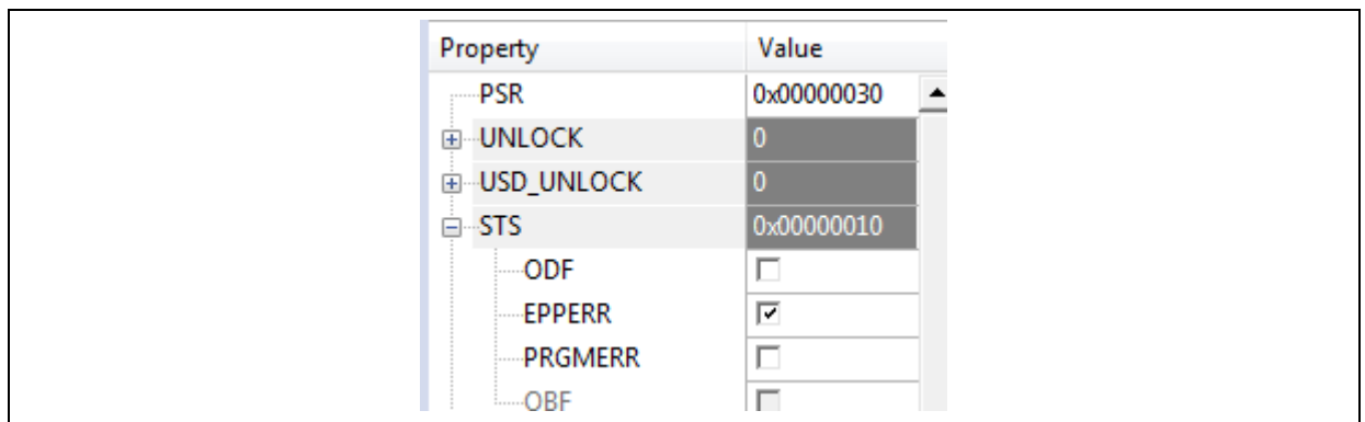
图 40. SLIB 写测试
