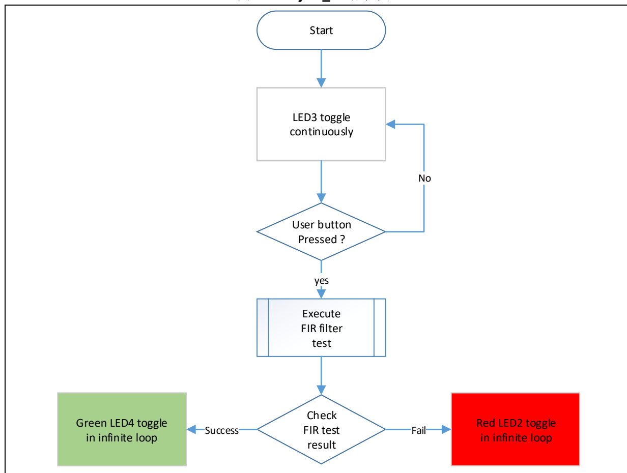
图 34. Project_L1 流程图
