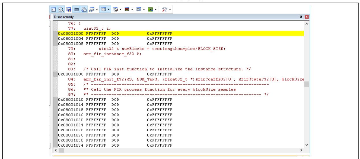
图 37. 代码查看
