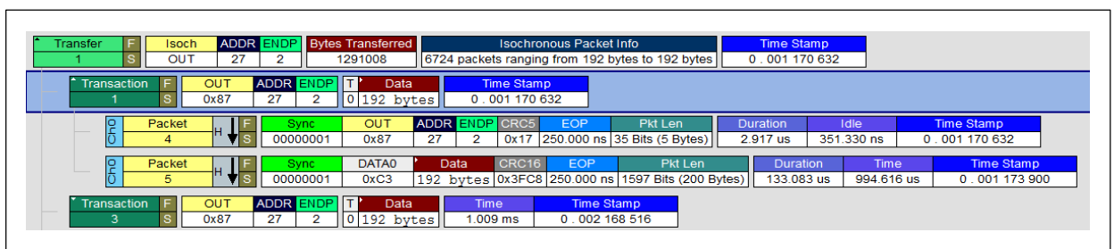
图 3. isochronous OUT 传输
