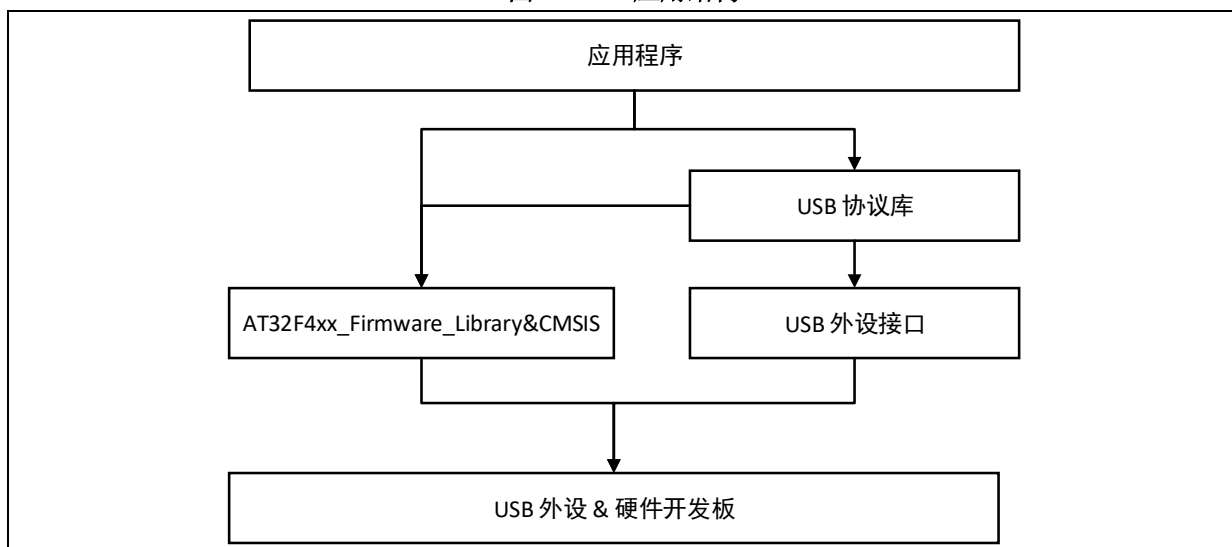
图 1. USB 应用结构
