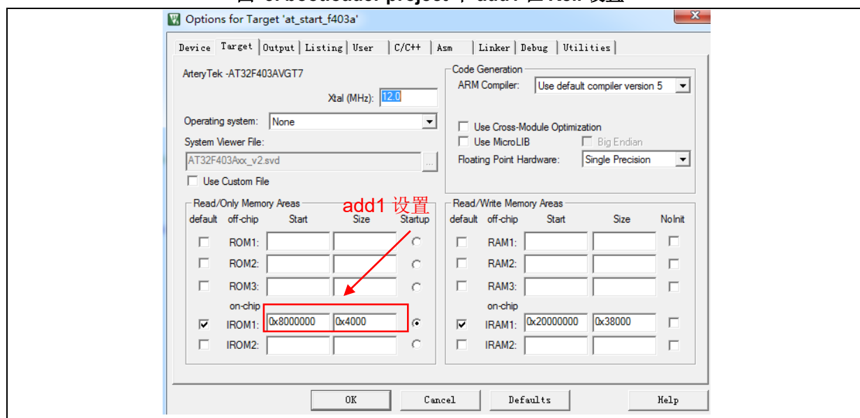
图 3. bootloader project 中 add1 在 Keil 设置
