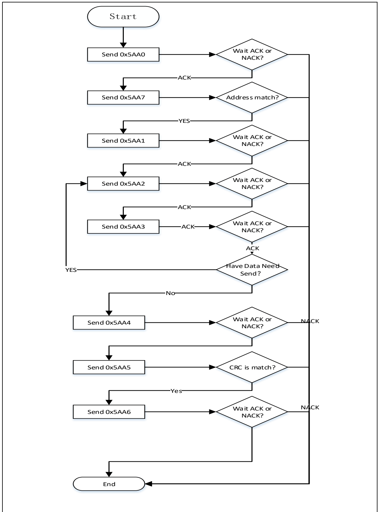
图 7. 上位机通信流程
