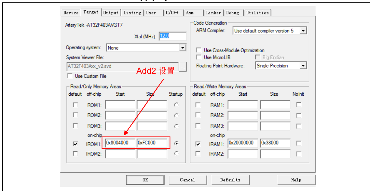
图 5. app project 中 add2 在 Keil 设置
