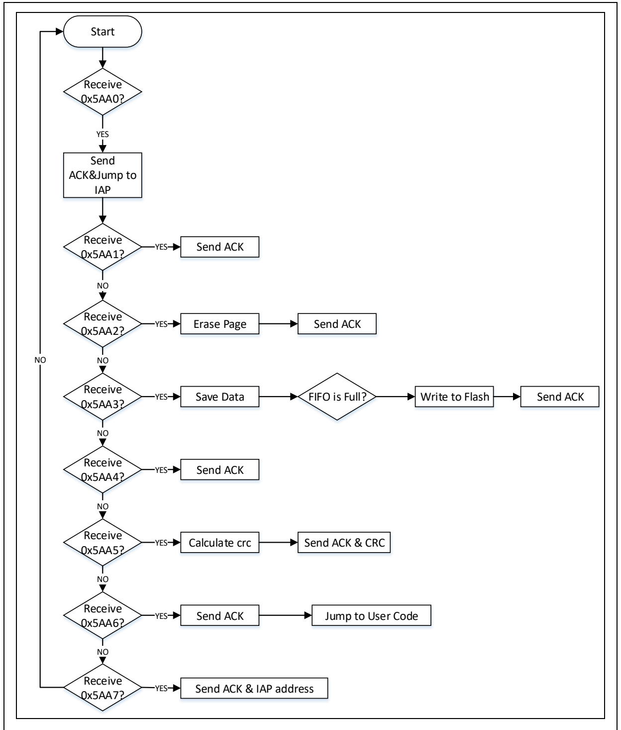
图 8. IAP 端下位机通信流程
