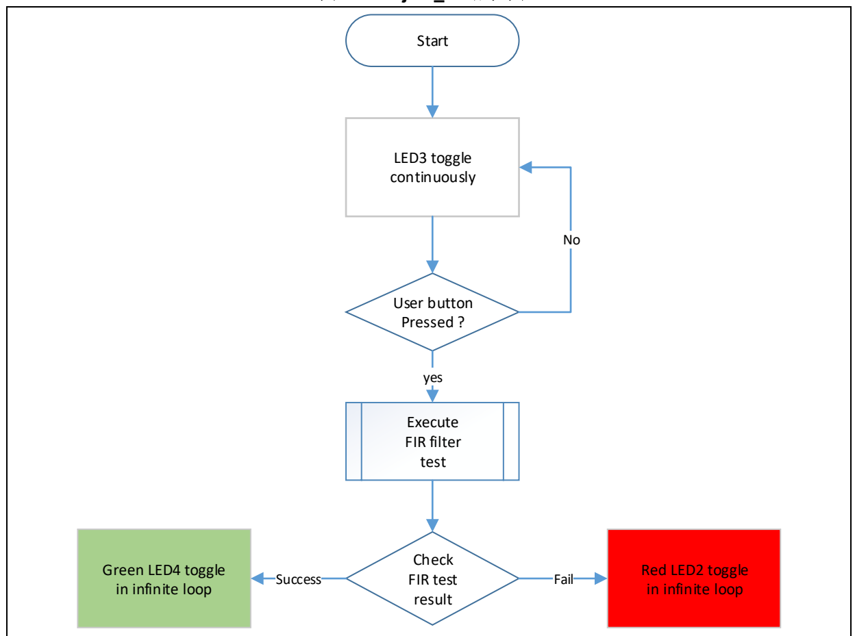
图 35. Project_L1 流程图
