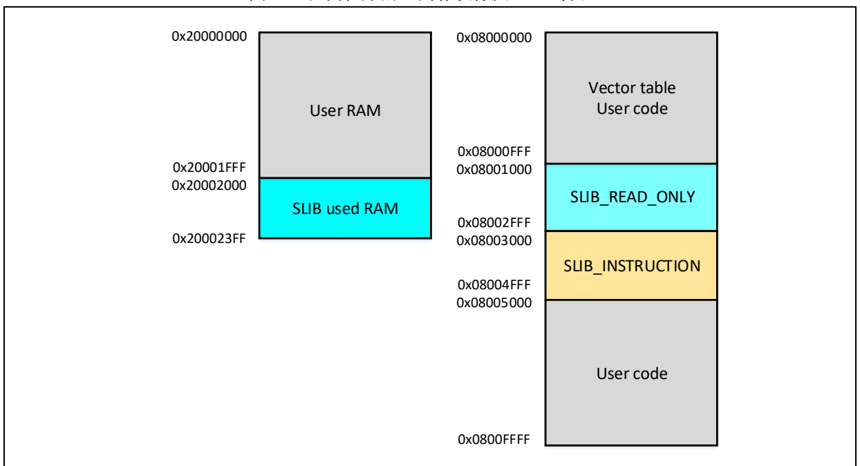
图 14. 范例程序的主闪存映像及 RAM 分区
